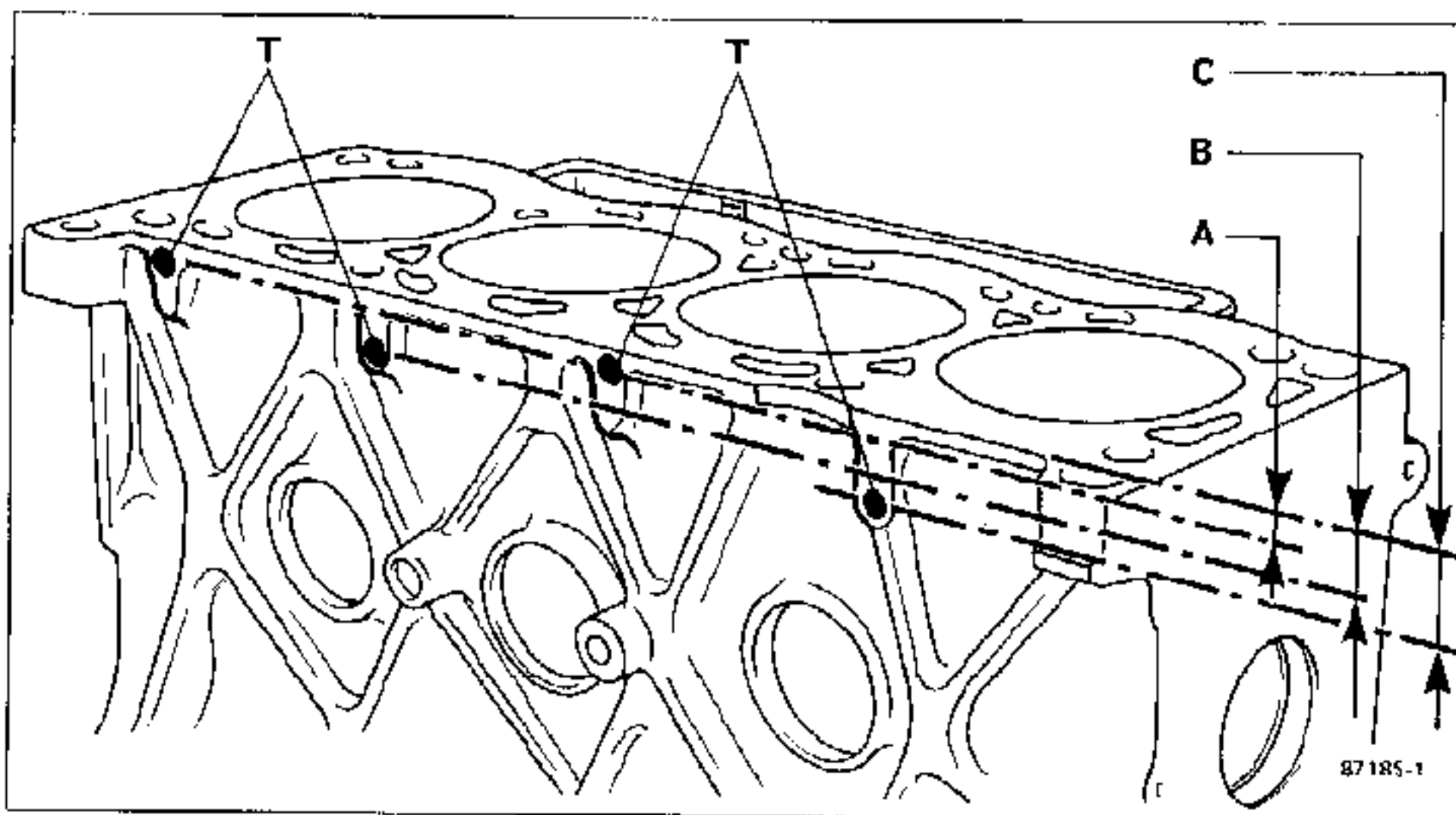
Position du trou T
